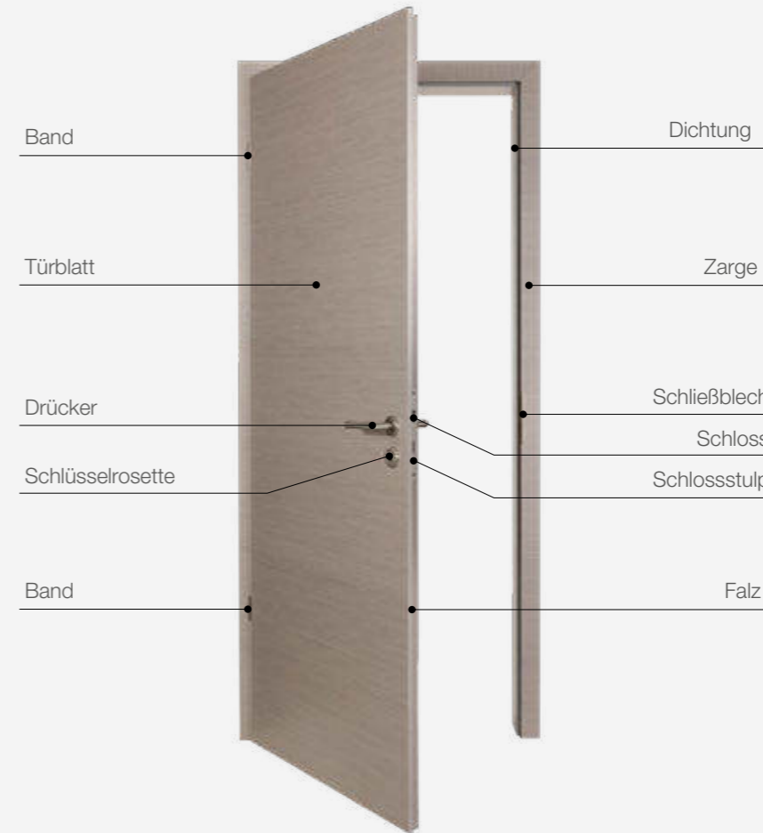
Türseite Bandseite Futterseite Bandgegenseite
